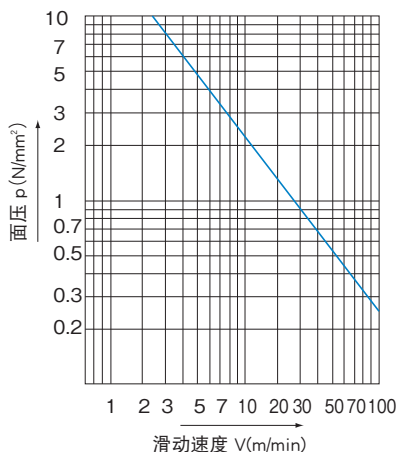
图1 pV值
